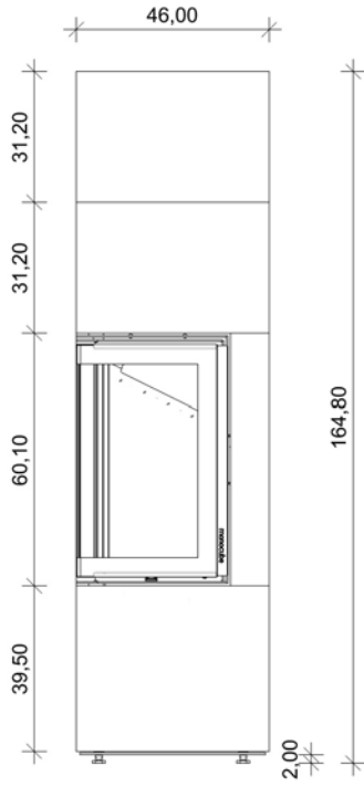
Ansicht Vorderseite
